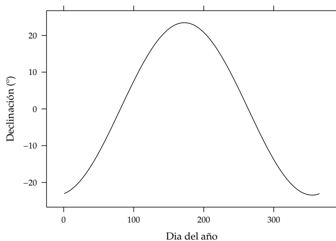
FIGURA 2.2: Declinación.
