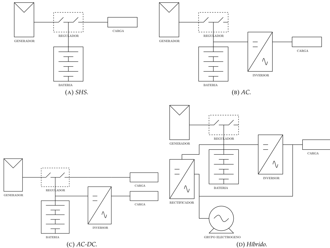
FIGURA 7.1: Configuraciones típicas.
