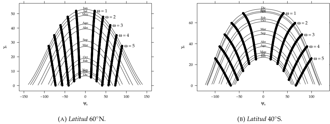
FIGURA 2.9: Diagrama de trayectoria solar según los ángulos de elevación y acimut en dos localidades terrestres.
