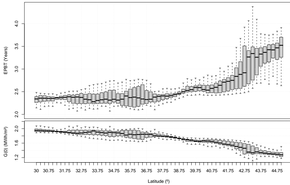
FIGURA 10.1: EPBT de un SFCR con seguimiento a doble eje para la región geográfica comprendida entre -10^\circ y 10^\circ de longitud, y 30^\circ a 45^\circ de latitud. La figura inferior muestra los valores anuales de radiación global en el plano horizontal como referencia.
