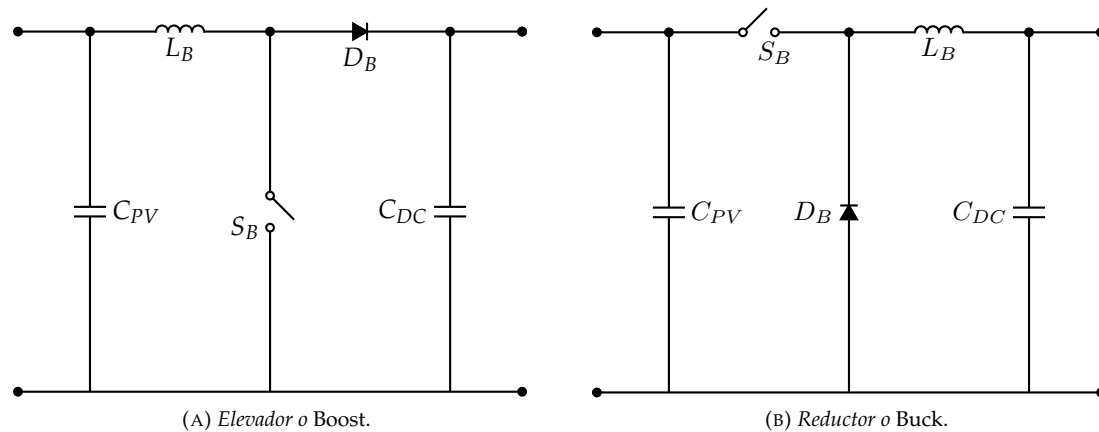
FIGURA 8.5: Convertidores DC-DC.
