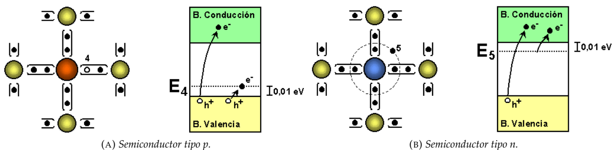
FIGURA 4.1: Semiconductores dopados.
