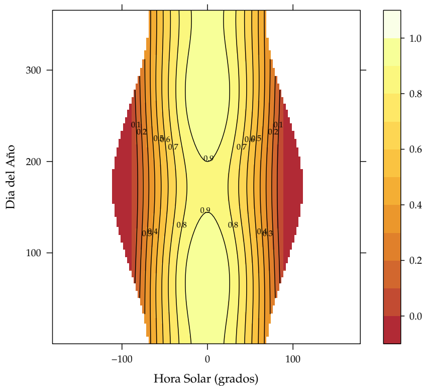
FIGURA 2.13: Coseno del ángulo de incidencia en un sistema estático a lo largo del día y año para un sitio con latitud 40°N.
