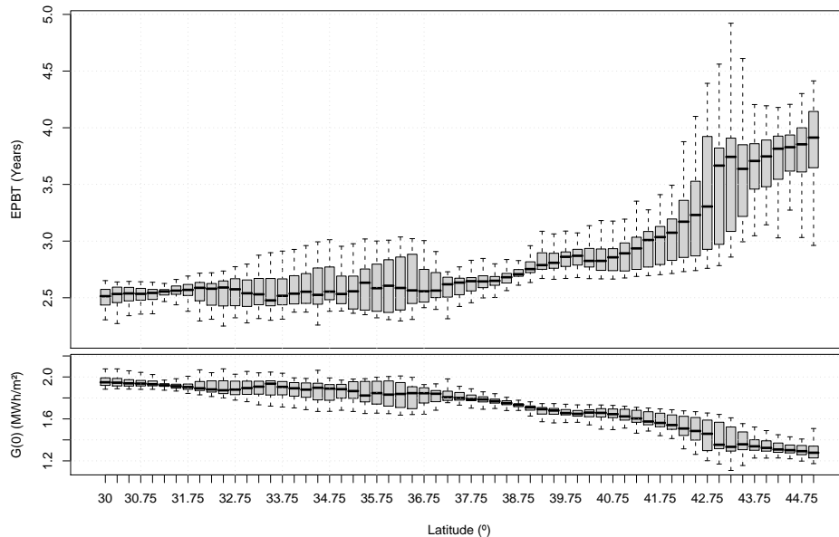
FIGURA 10.2: EPBT de un SFCR con seguimiento horizontal N-S para la región geográfica comprendida entre -10^\circ y 10^\circ de longitud, y 30^\circ a 45^\circ de latitud. La figura inferior muestra los valores anuales de radiación global en el plano horizontal como referencia.
