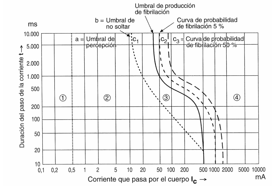
FIGURA 9.1: Efecto de la corriente que circula por el cuerpo humano según su intensidad y tiempo de duración [PG00b; PG00a].
